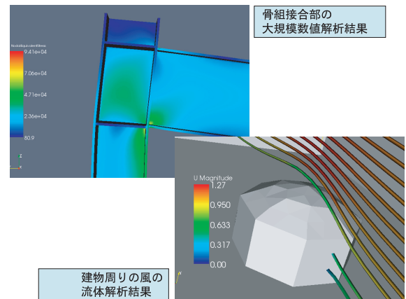
コンピュータによる解析
