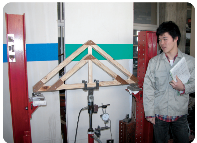
建築構造実験
