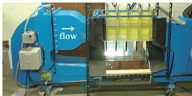
魚道に関する遡上実験
