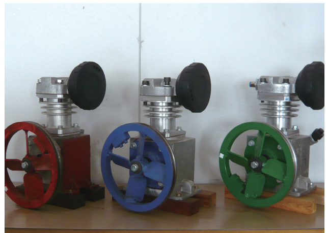
創生工学実習作品（小型空気圧縮機）
