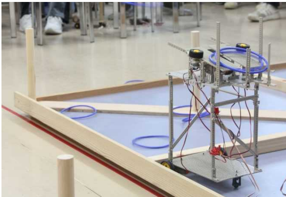
写真は昨年度の岐阜地区予選大会で優勝したロボットです。
