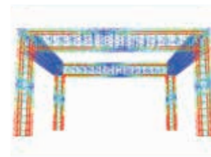
鉄筋コンクリート造骨組の精密解析
