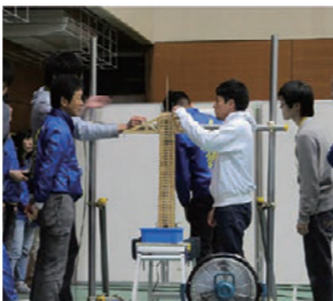
全国高专デザインコンペティション(課題の木製タワーを振動台に設置)
