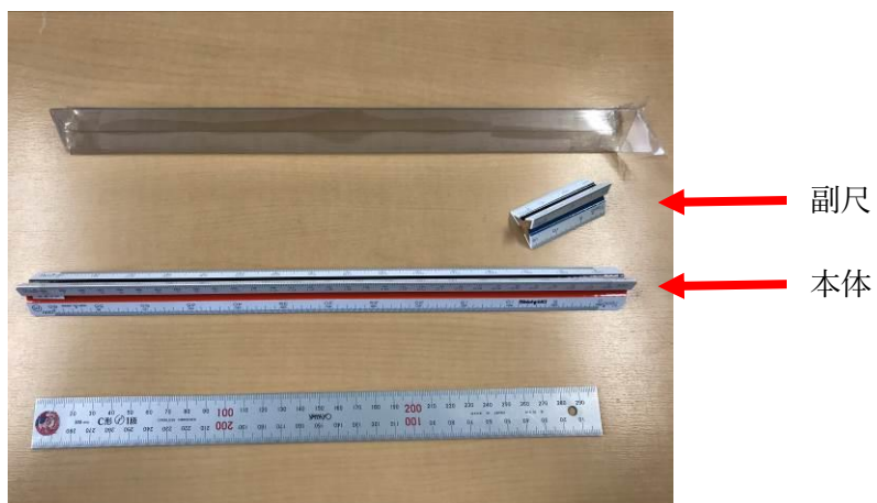
三角スケール
