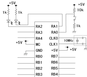
図 3.1 ライントレーサ用 PIC 回路
