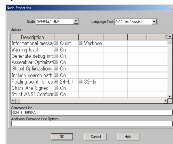
図 2.3 コンパイルオプション
