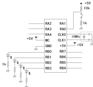
図 1.1 LED 点灯用 PIC 回路
