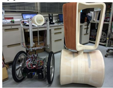
ツアーガイドロボットの試作
