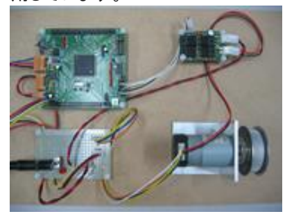
DC モータ制御実験装置
